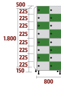
FZP-40/2 COD: 53586 108kg · 0,72m 3
