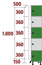
FPP-30/1 COD: 53551 40kg · 0,28m 3
