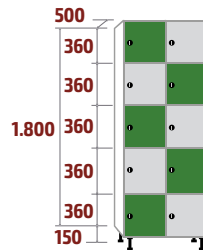
FPP-40/2 COD: 53566 88kg · 0,72m 3
