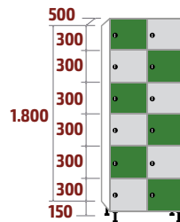
FBP-40/2 COD: 53576 94kg · 0,72m 3
