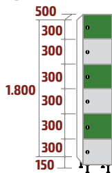
FBP-30/1 COD: 53561 42kg · 0,28m 3
